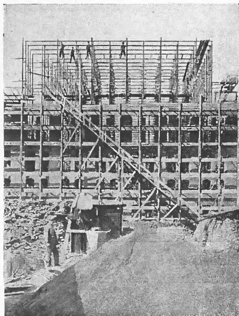
Bibliothèque à 10 étages, avec planchers métalliques. Vue prise en cours de construction. Hauteur des étages 2 m 20.
