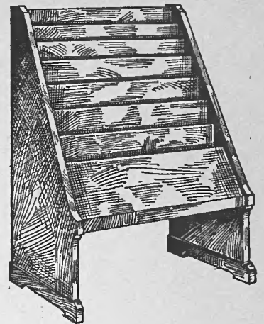
MEUBLE A PÉRIODIQUES sans tiroirs
