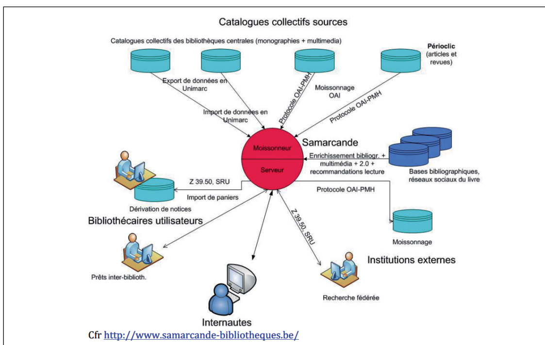
Architecture de l'interface dans le SID
