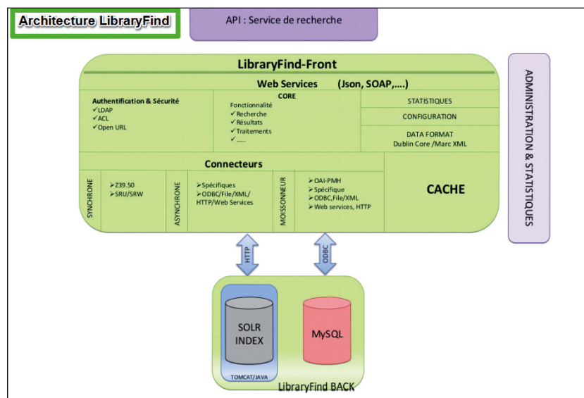
Architecture de l'interface dans le SID
