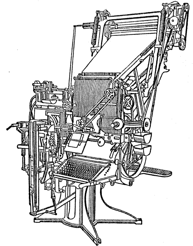
Fig. 17 La linotype de Mergenthaler, 1884
