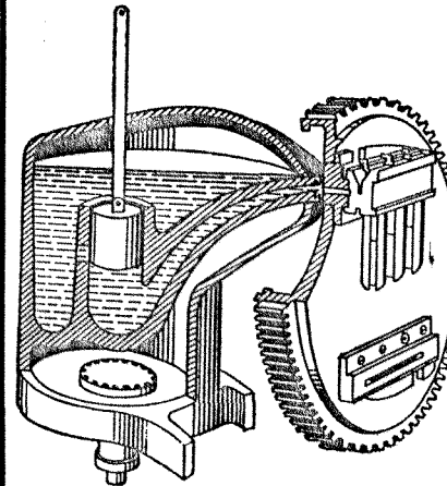
Fig. 18 Détail de la fondeuse de la linotype Une enceinte, chauffée par un brûleur à gaz, contient le métal fondu, à gauche. L'action d'une pompe envoie le métal dans la ligne composée de matrices portée par la roue de droite. La rotation d'un demi-tour de la roue met en place le moule placé à sa partie inférieure sur la figure et qui va recevoir une nouvelle ligne de matrices, pendant que la précédente est évacuée.
