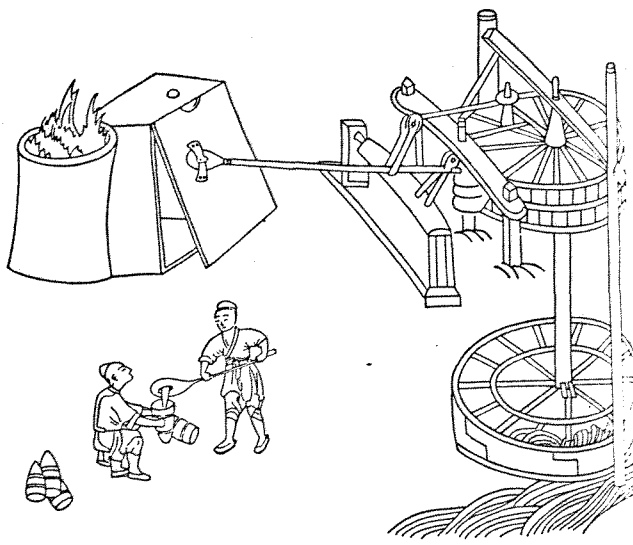
FIG. 2. — SOUFFLET HYDRAULIQUE POUR LES FOURNEAUX MÉTALLURGIQUES (1313). (D'après J. Needham.)
