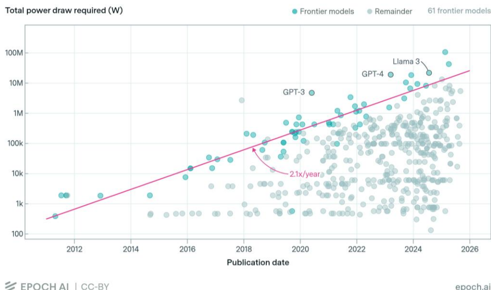
Figure 12 - Puissance de calcul requise estimée pour entraîner les modèles d'IA. Source : Epoch AI
